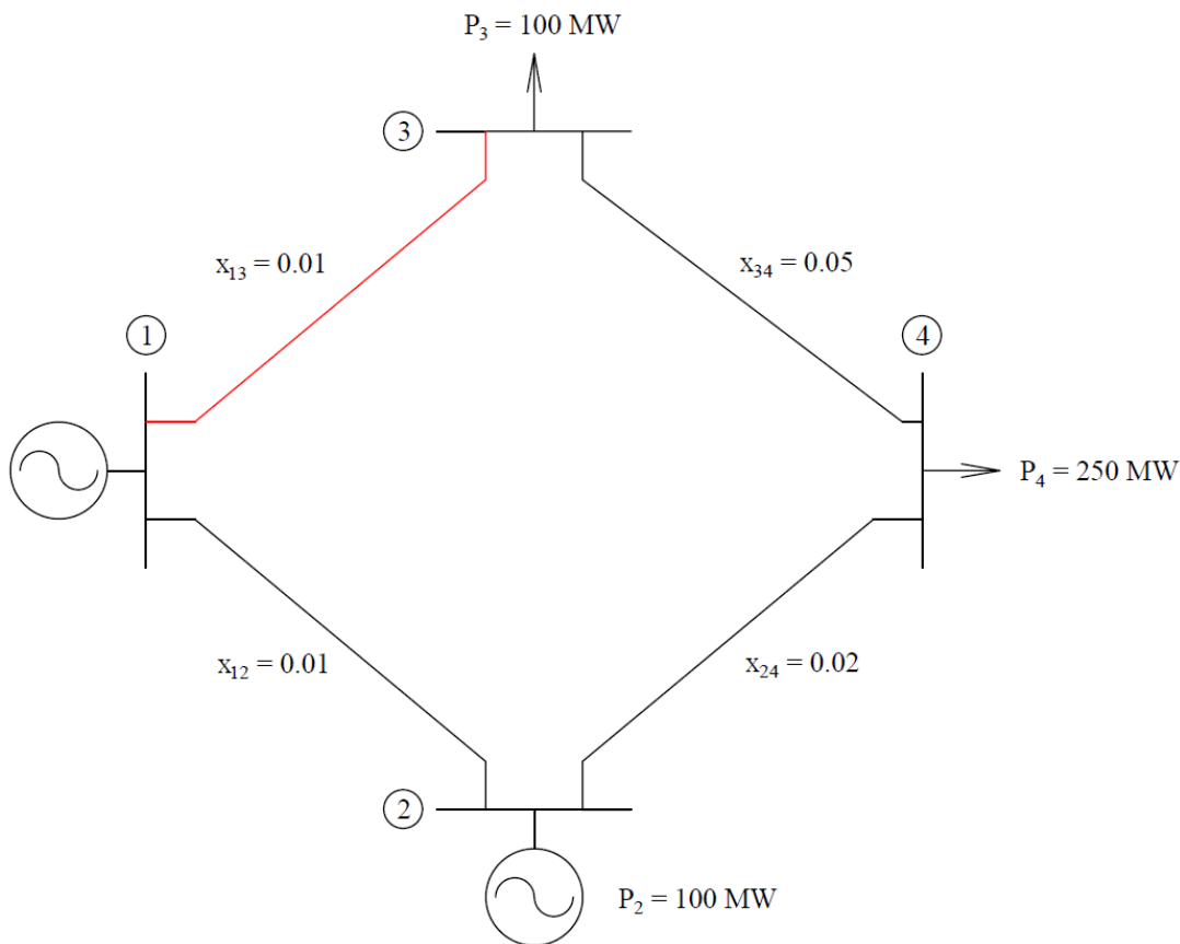
Slika 3. Jednopolna šema elektroenergetskog sistema
