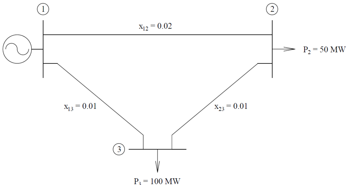
Slika 1. Jednopolna šema elektroenergetskog sistema
