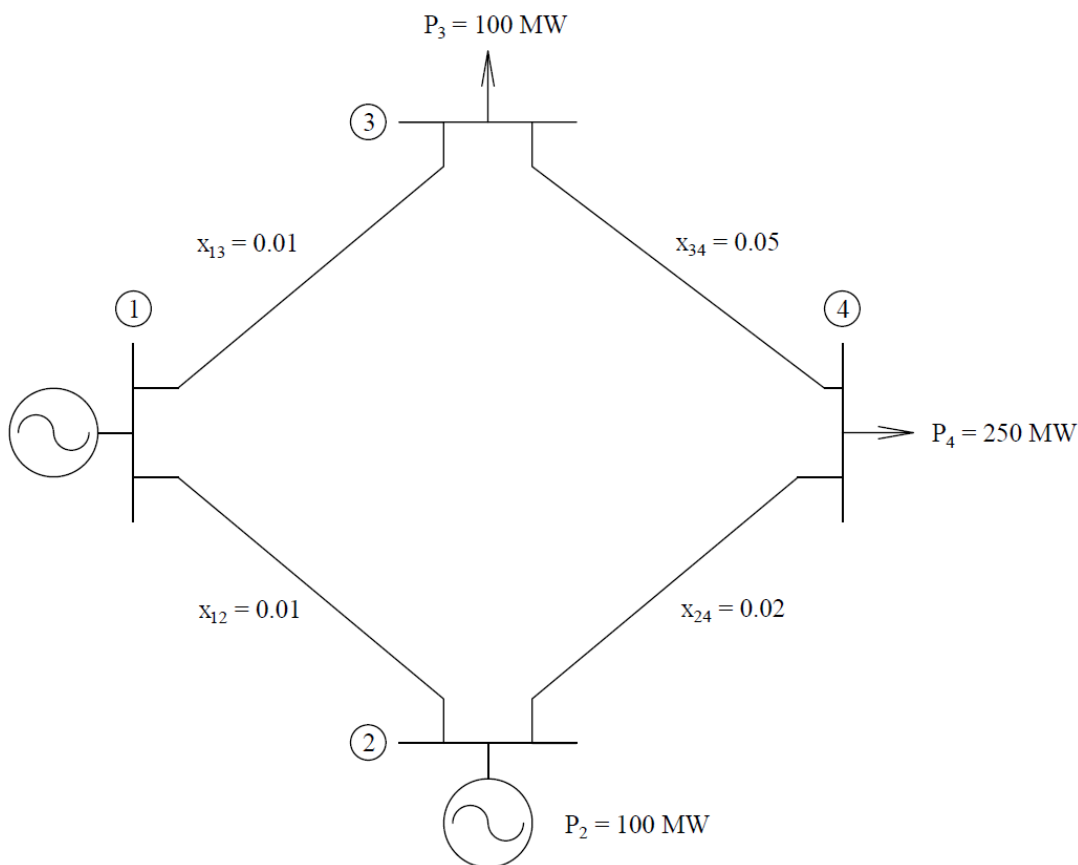
Slika 2. Jednopolna šema elektroenergetskog sistema
